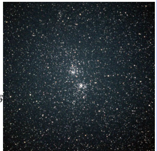
ペルセウス座二重星団 NGC869 NGC884
